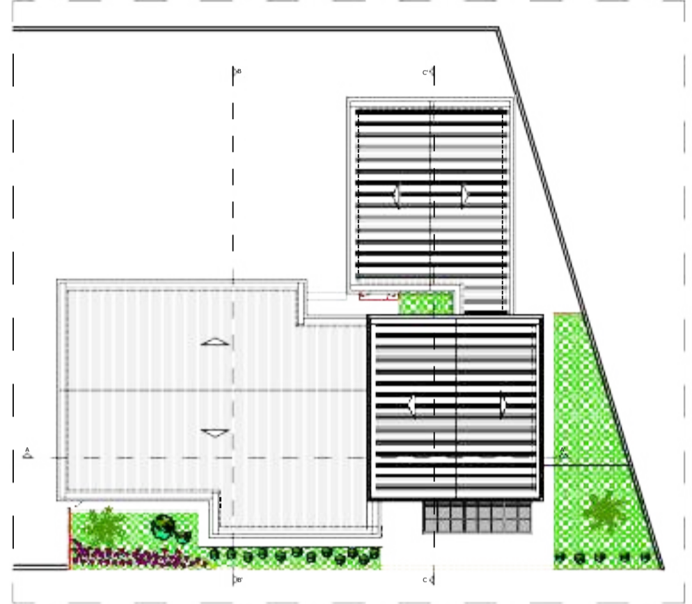
Planta de Cobertura Escala 1/150
