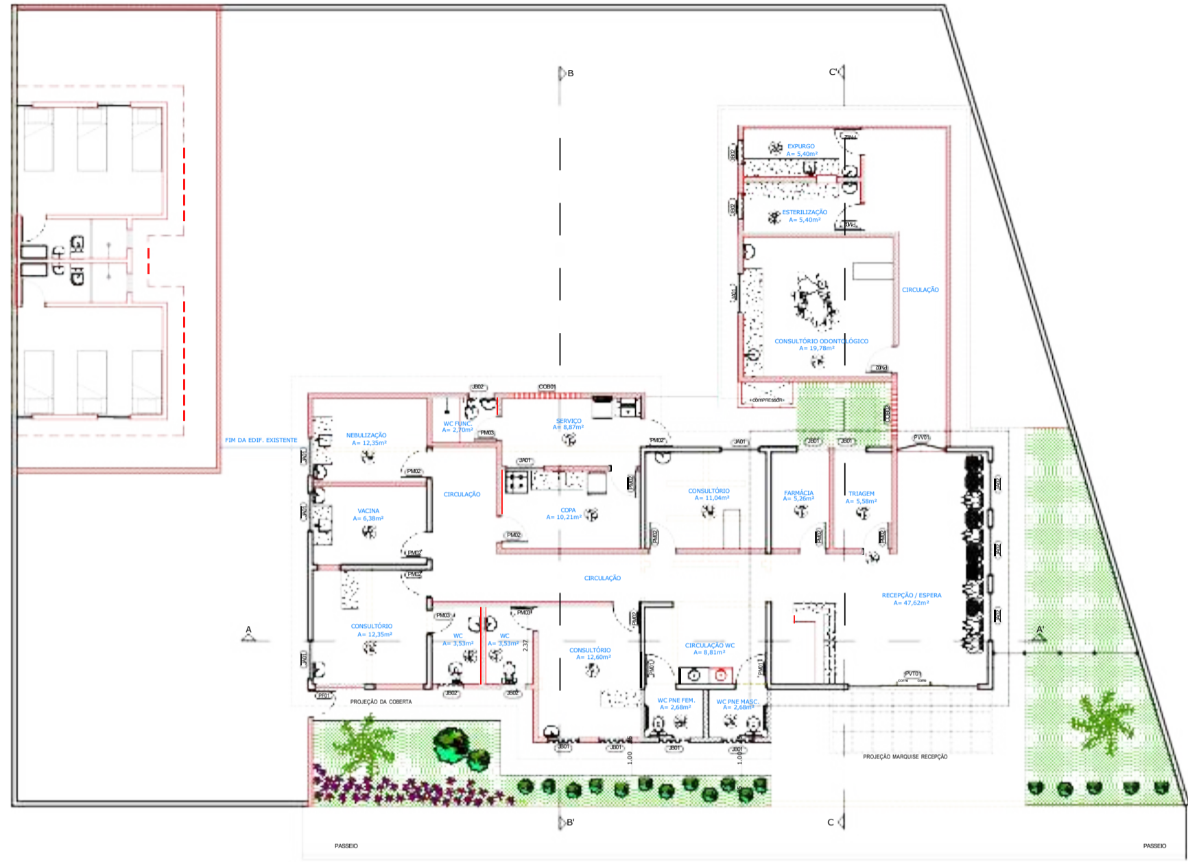
Planta Baixa Construir / Demolir Escala 1/100
